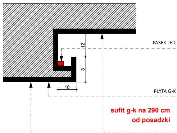
DETAL, PRZEKRÓJ B-B
