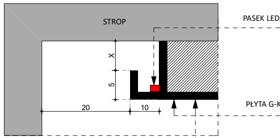
DETAL, PRZEKRÓJ A-A
